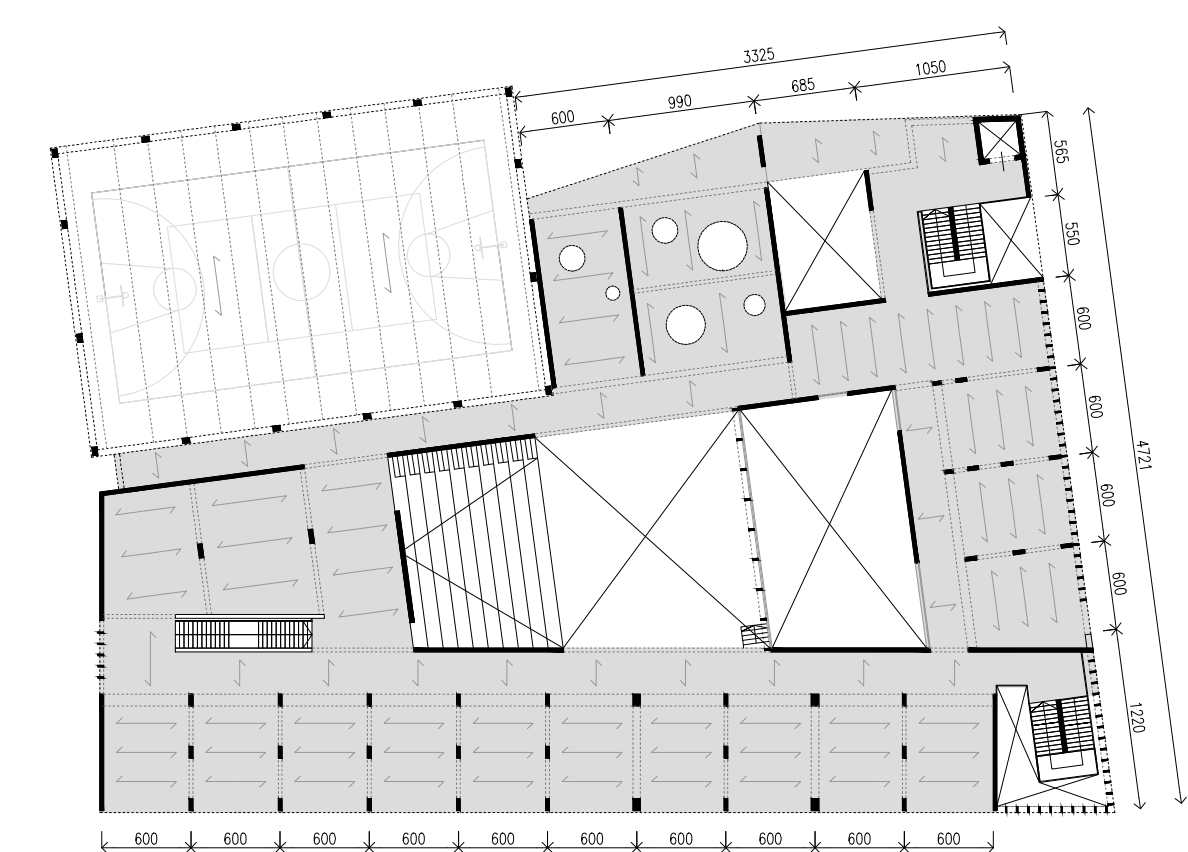
SCHEMA STRUTTURE: PRIMO IMPALCATO scala 1:500
